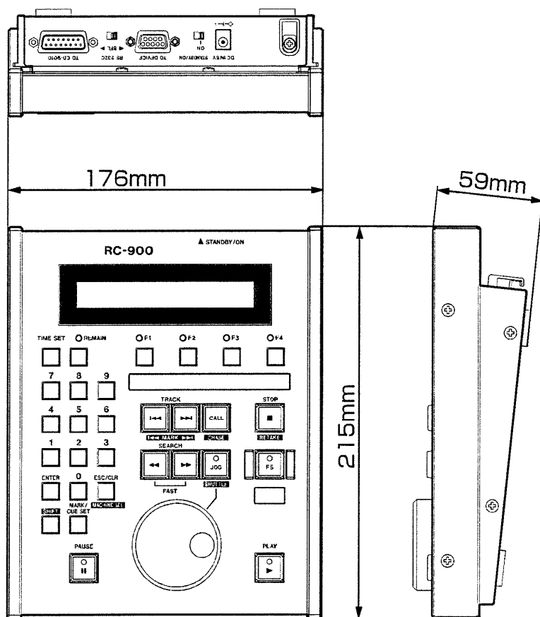
[寸法図]
